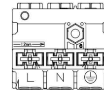
端子台 (20A-300V)
