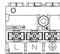
端子台 (20A-300V)
