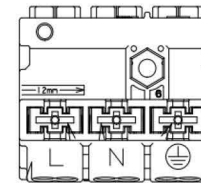
端子台 (20A-300V)
